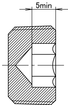
断面図 A-A
