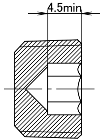
断面図 A-A
