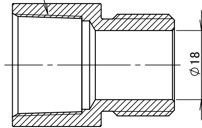
断面図 A-A
